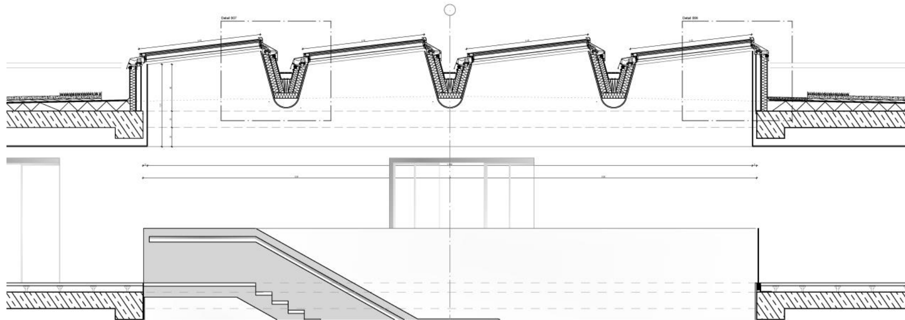
Schnitt AA
